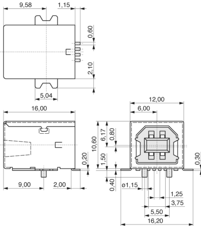
USB B, Buchse
