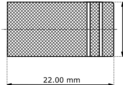
Gehäusehülse case sleeve
